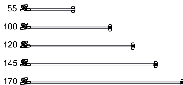
Lengder støttestag/ Lengths support brace
