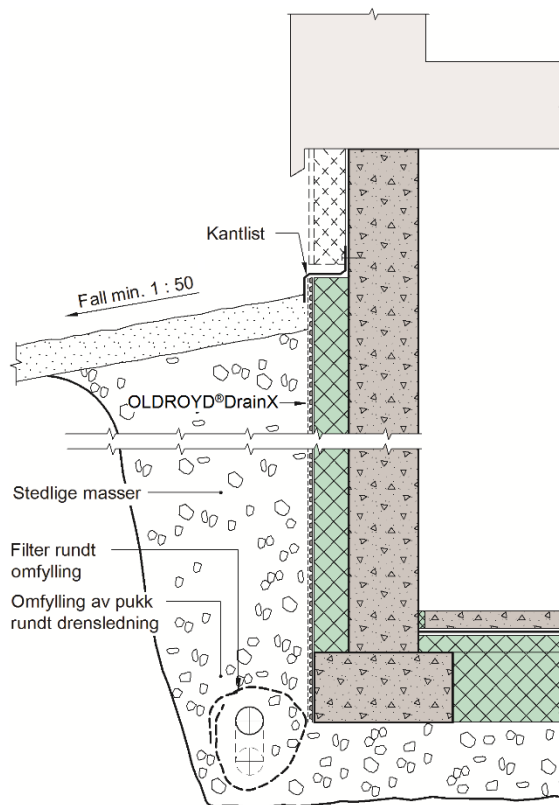
Fig. 3 Eksempel på bruk av OLDROYD® DrainX produktene på yttervegg mot terreng i oppvarmet kjeller
